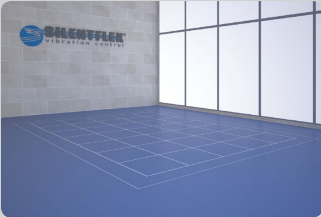
Sobre el foso se posicionan los apoyos nivelados (opcional) y se cubre el perímetro con lana de roca
